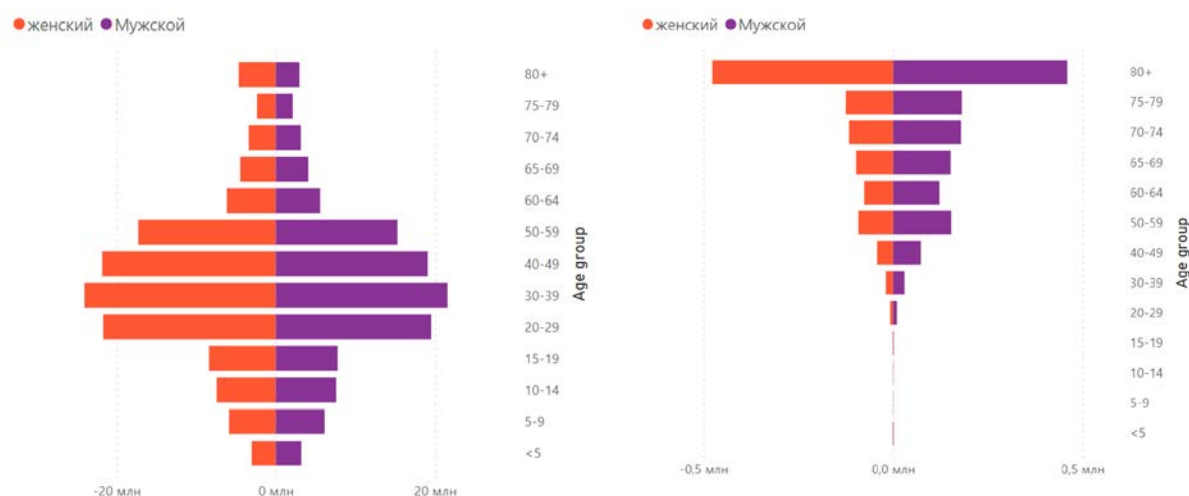
Рис. 3. Распределение по полу и возрастным группам числа заболеваний и летальных исходов вследствие COVID-19 в мире с 30.12.2019 по 02.05.2022, чел. [10]
